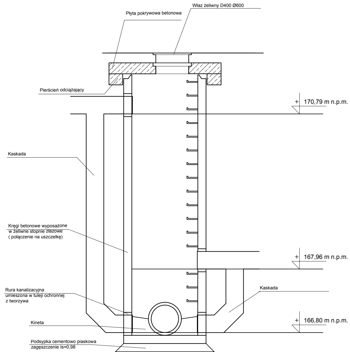
Studnia betonowa S1
